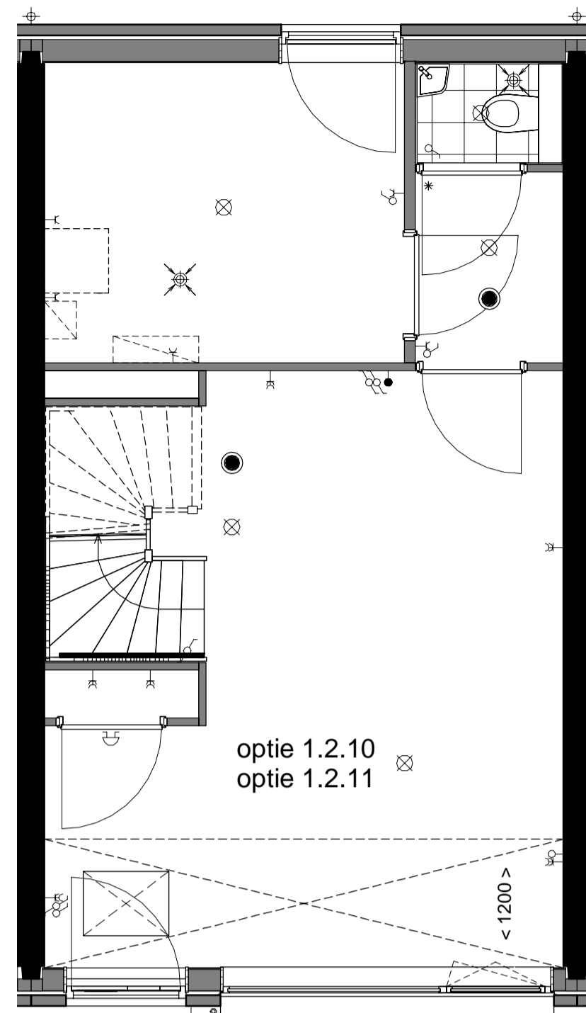
begane grond
