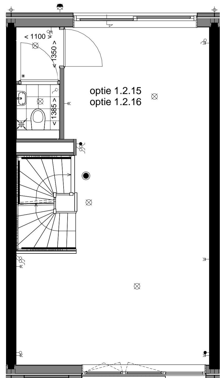
1e verdieping
